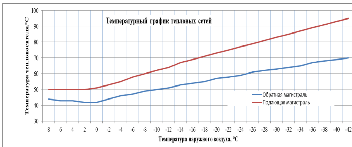
Рисунок 2 – Температурный график котельной
